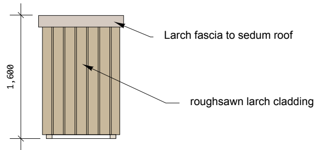
Elevation 1:50
